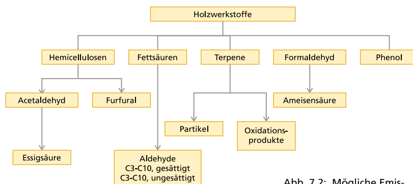
Abb. 7.2: Mögliche Emissionen organischer Verbindungen aus Holzwerkstoffen
