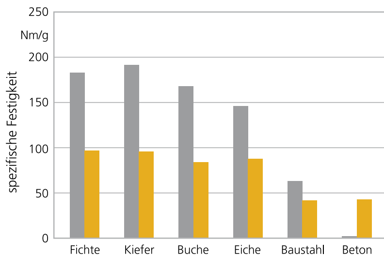
Abb. 2.3: Spezifische Zugfestigkeit (grau) und Druckfestigkeit (gelb) von einheimischen Hölzern im Vergleich zu Baustahl und Hochleistungsbeton
