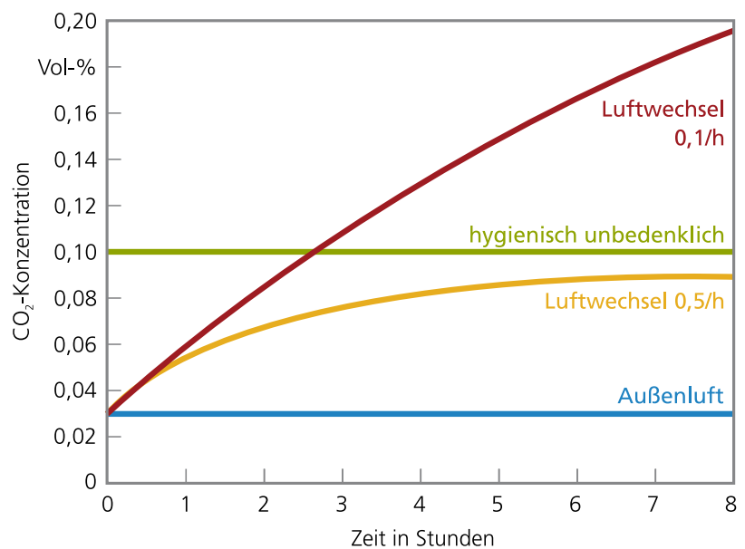
Abb. 6.1: Zunahme der CO 2 -Konzentration in einem 50 m 3 Raum durch eine ruhende Person bei verschiedenen Luftwechselraten
